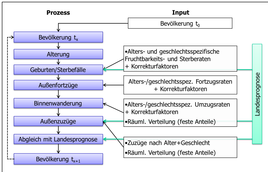
Abb. 8: Grundstruktur Simulationsmodell Bevölkerungsentwicklung
